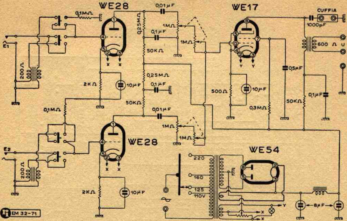
Preamplificatore portatile PP/2 a 2 ingressi
