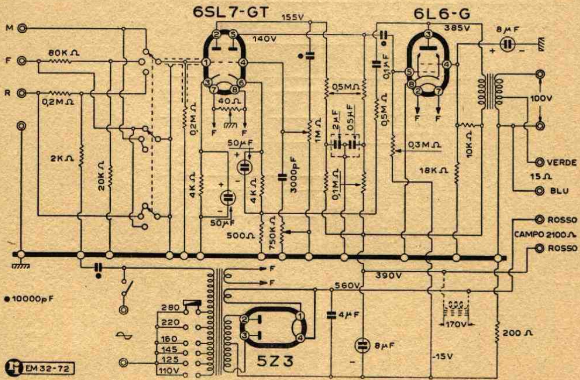
Amplificatore mod. ELA 515
